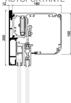
PORTERIA BÁSICA AUTOPORTANTE
